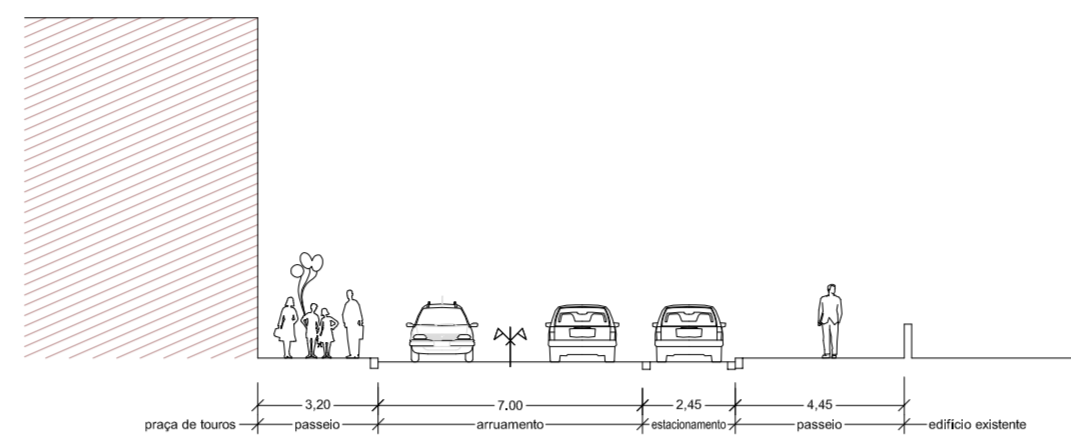
PERFIL TRANSVERSAL TIPO 2
